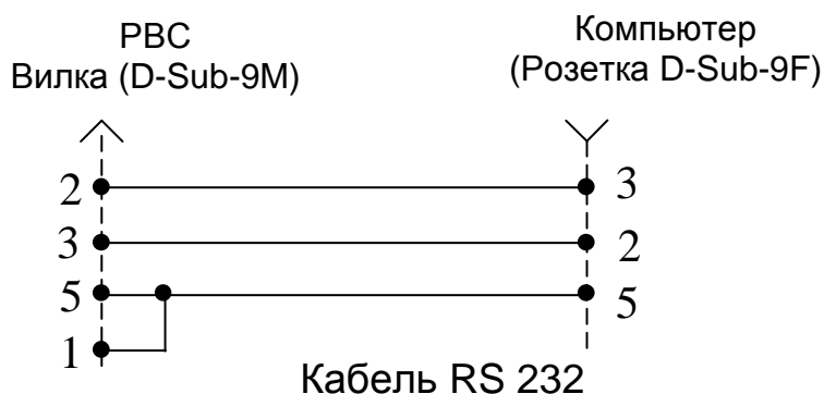
Цепи сопряжения радиостанции с компьютером
