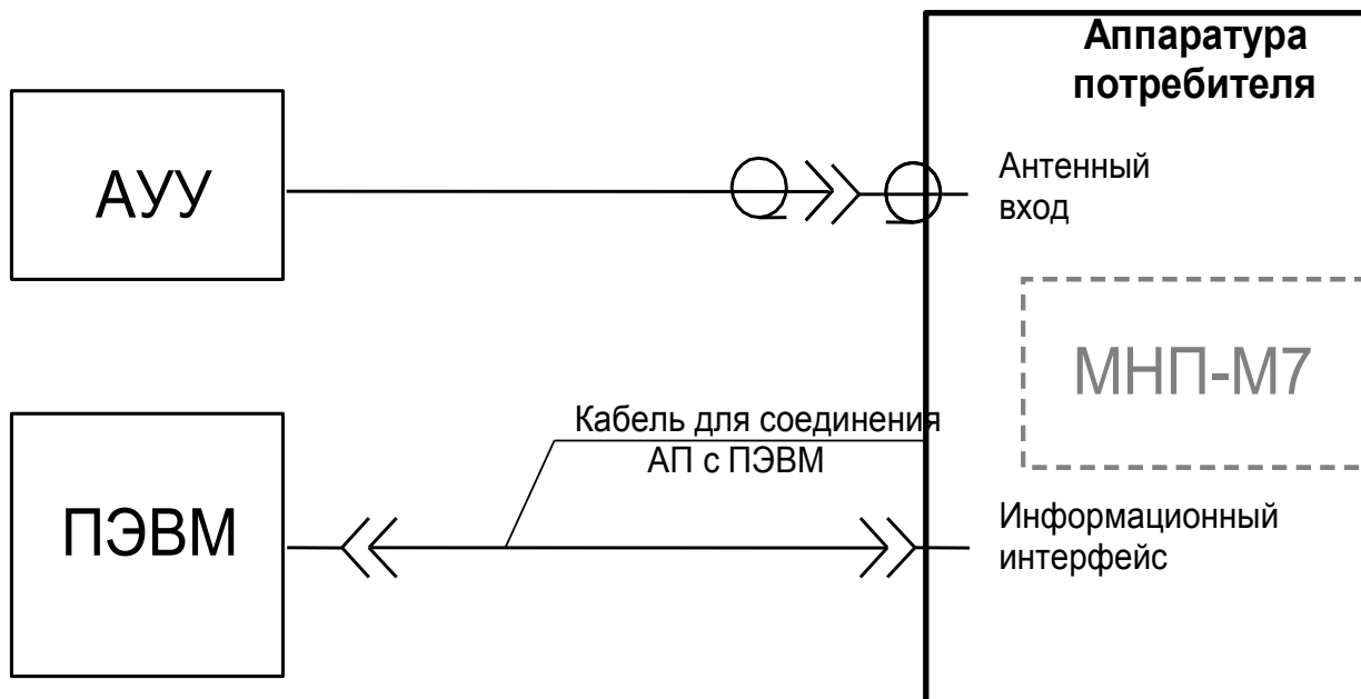
Рисунок 9 – Схема подключения МНП-М7 при работе по реальному сигналу
