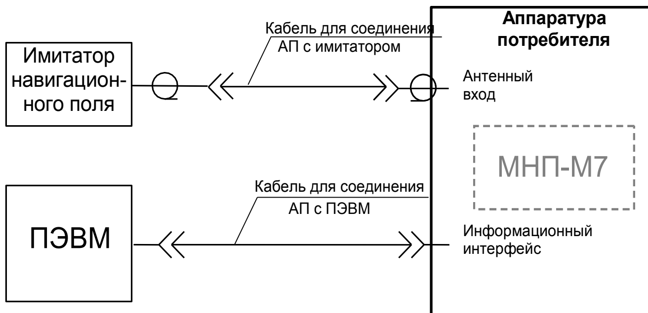
Рисунок 10 – Схема подключения МНП-М7 при работе с имитатором навигационного поля
