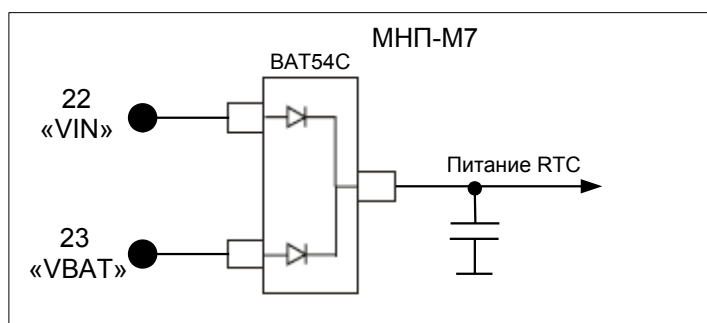
Рисунок 2 — Питание RTC в МНП-М7
