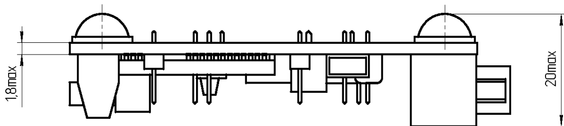
Рисунок Б.2 – Габаритный чертеж средства отладочного ЦВИЯ.468219.015-01
