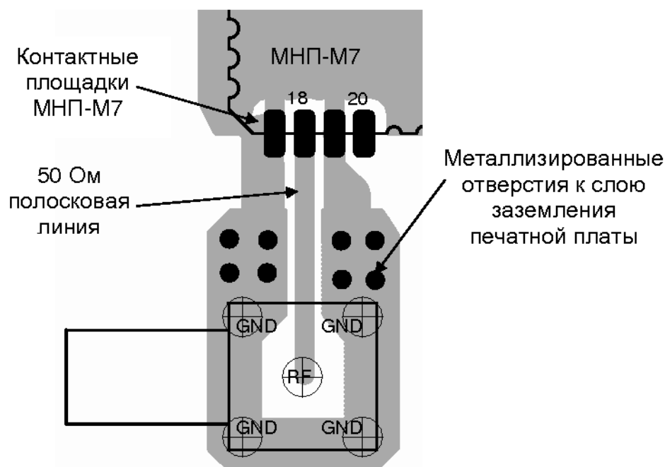
Рисунок 8 – Подключение ВЧ-соединителя к приемнику
