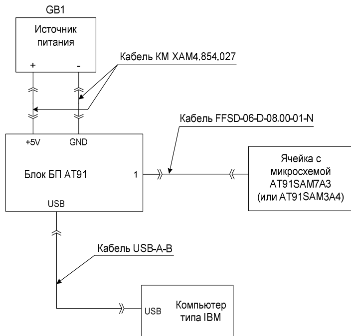
Рисунок 2.1 – Схема рабочего места
