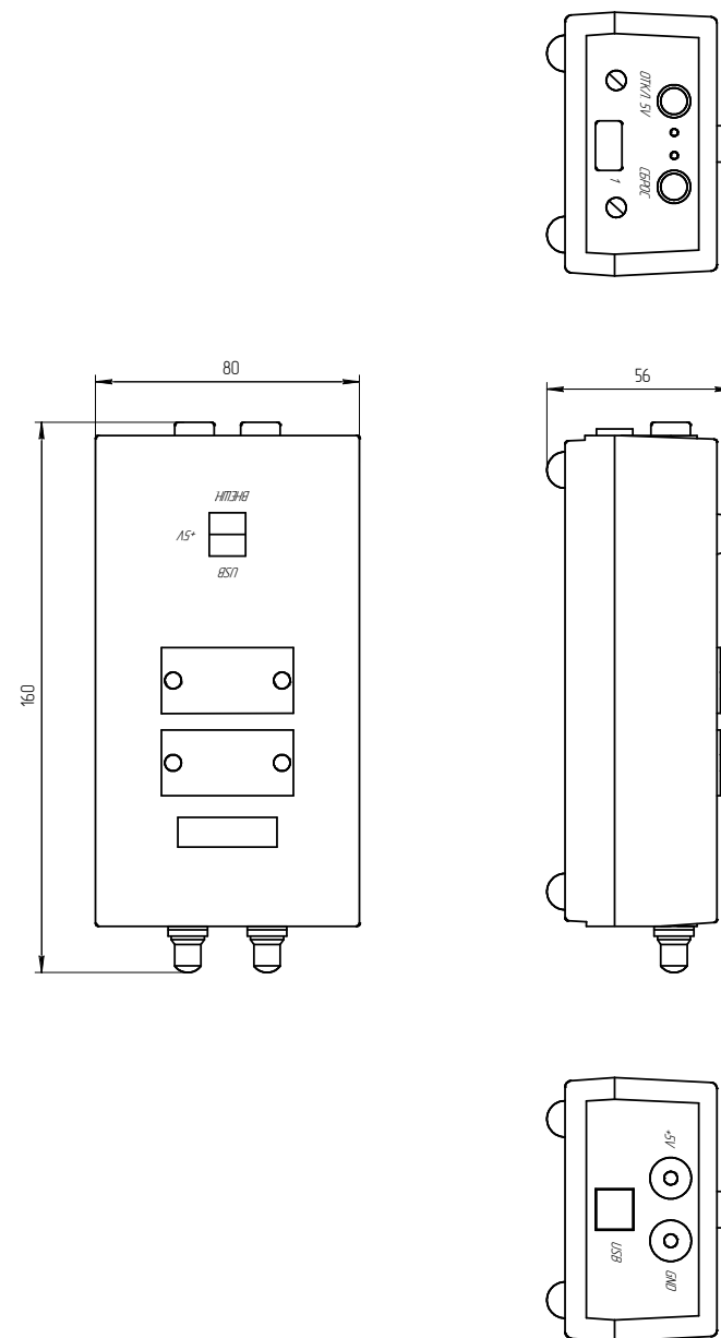
Рисунок 1.1 - Внешний вид блока БП АТ91
