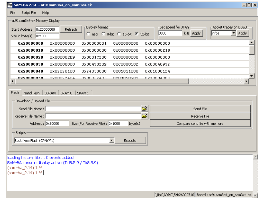
Рисунок 2.14 – Рабочее окно программы
