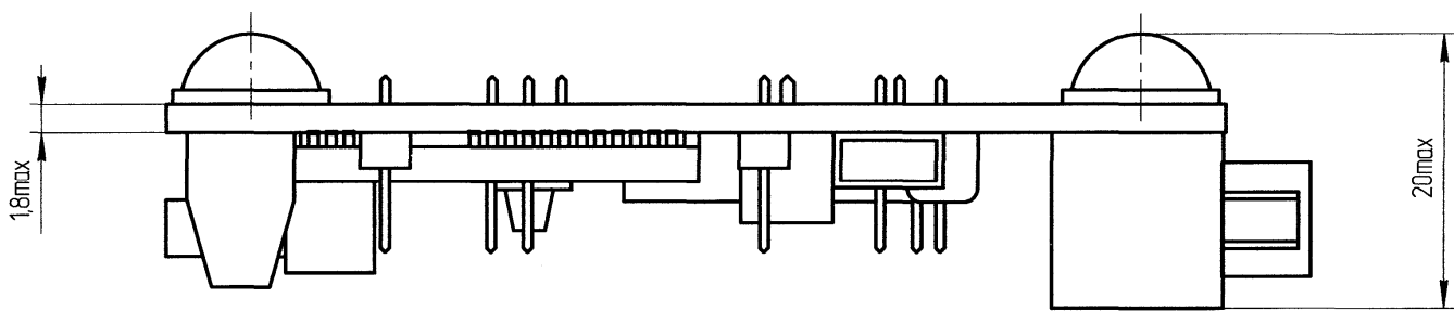
Рисунок Б.1 – Габаритный чертеж средства отладочного ЦВИЯ.468219.015-02
